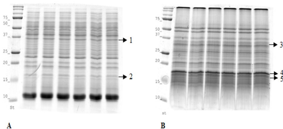
Figura 1.- Geles teñidos con Coomassie. A; Fracción hidrosoluble. Las bandas indicadas son (1) Pap s 34 KD y (2) Pap s 17 KD. B; Fracción liposoluble. Las bandas indicadas son (3) caleosina, (4) oleosina y (5) ArgJ. Los marcadores moleculares están indicados.
