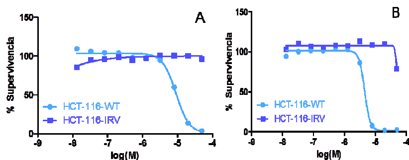
Figura 2.- Citotoxicidad de Elisidepsin. (A) Incubación de 30min. (B) Incubación de 72h. Los resultados se expresan en porcentaje de supervivencia en comparación al control.
