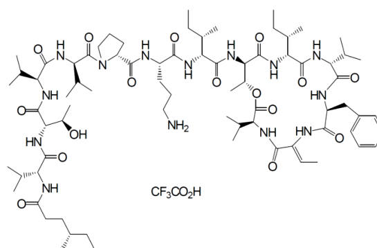
Figura 1.- Estructura química de Elisidepsin.
